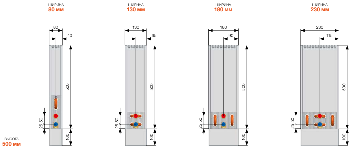
Высота стоек на чистый пол у всех моделей KORALINE 100 мм. Размеры указаны в мм. Технические изменения предусмотрены.
